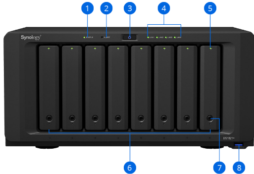
前面板
