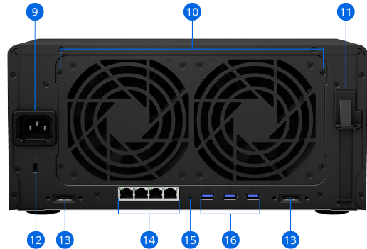
背面板
